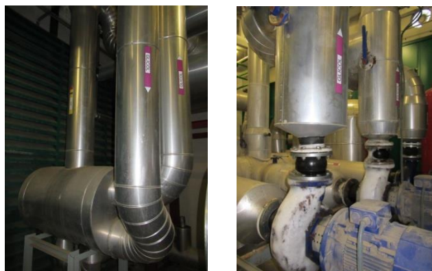
Intercambiador NH 3 /GLICOL y bombas de glicol ya refrigerado Foto: C. Artero
