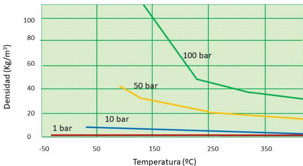
Densidad del amoníaco gas en función de la Tª y la Presión Fuente: Enginnering ToolBox. Ilustr. M. Albaladejo
