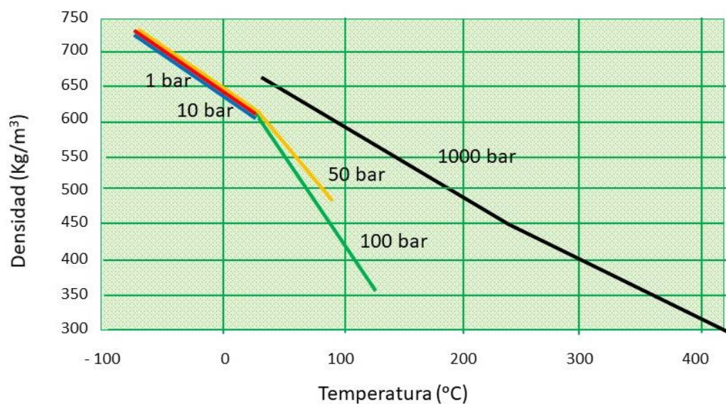
Densidad del amoníaco líquido en función de la Tª y la Presión Fuente: Enginering ToolBox. Ilustr. M. Albaladejo
