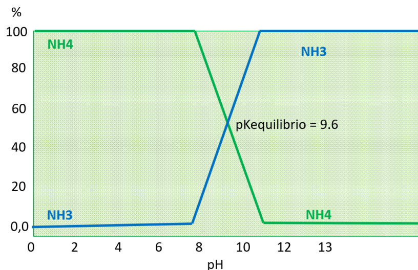
Valor de PH en función de la concentración de iones amonio
